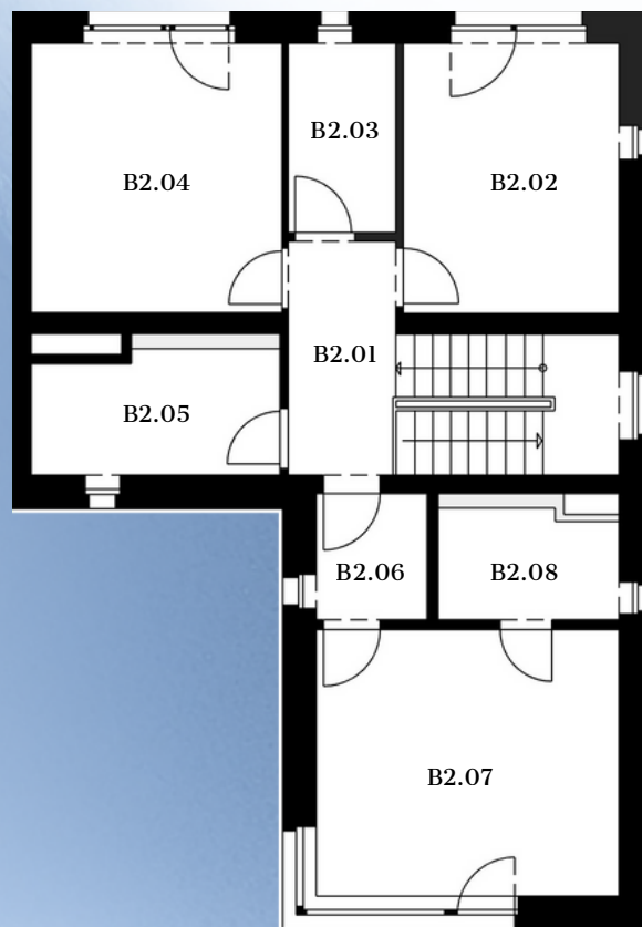
2.NP
